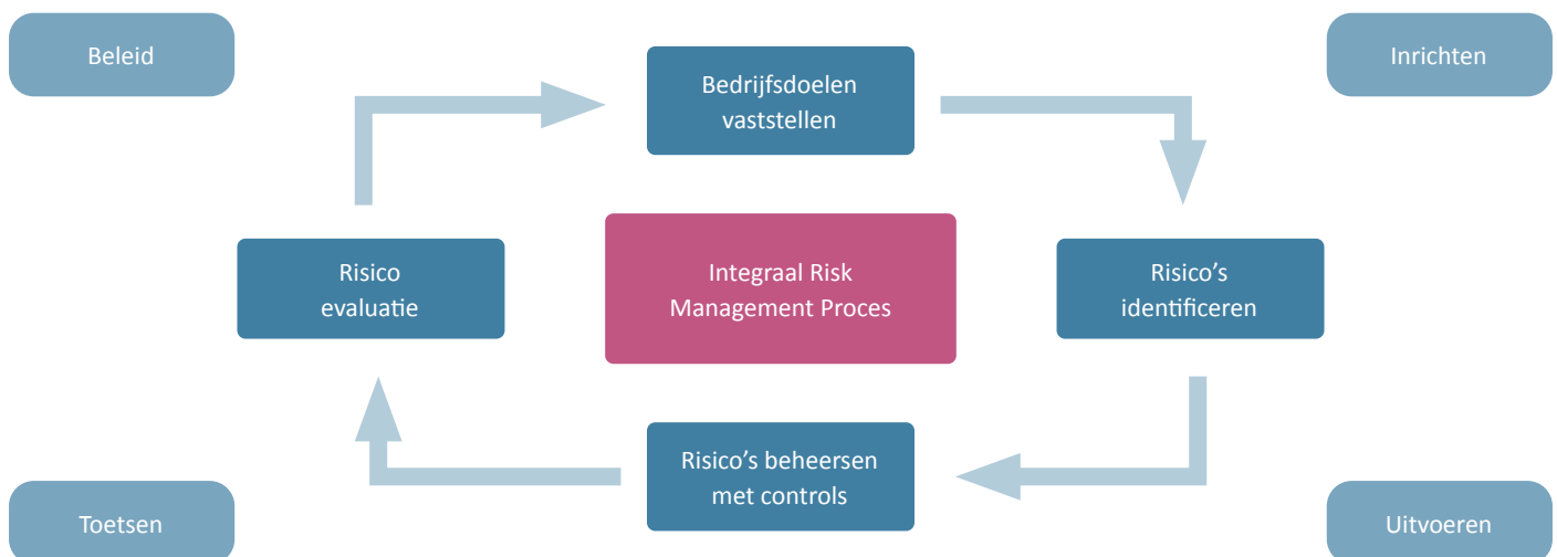
FIGUUR 3: RISICOMANAGEMENTCYCLUS
